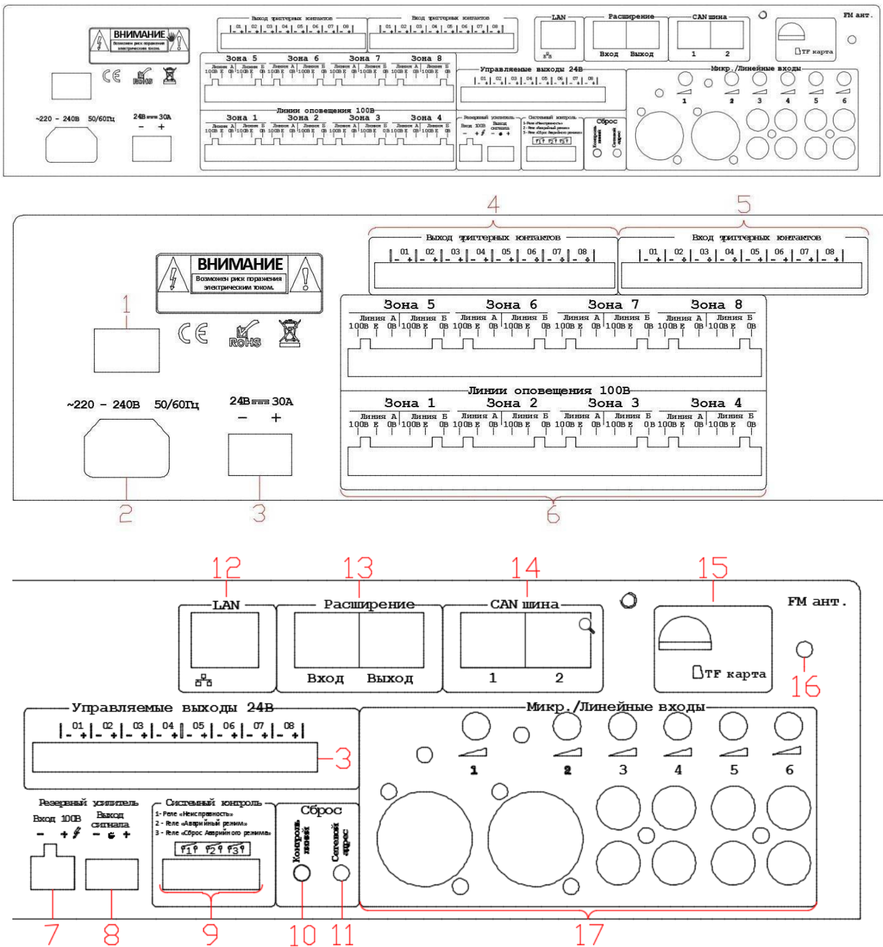
Рис. 1.1. Контроллер системы LPA-DUO-M (задняя панель)
